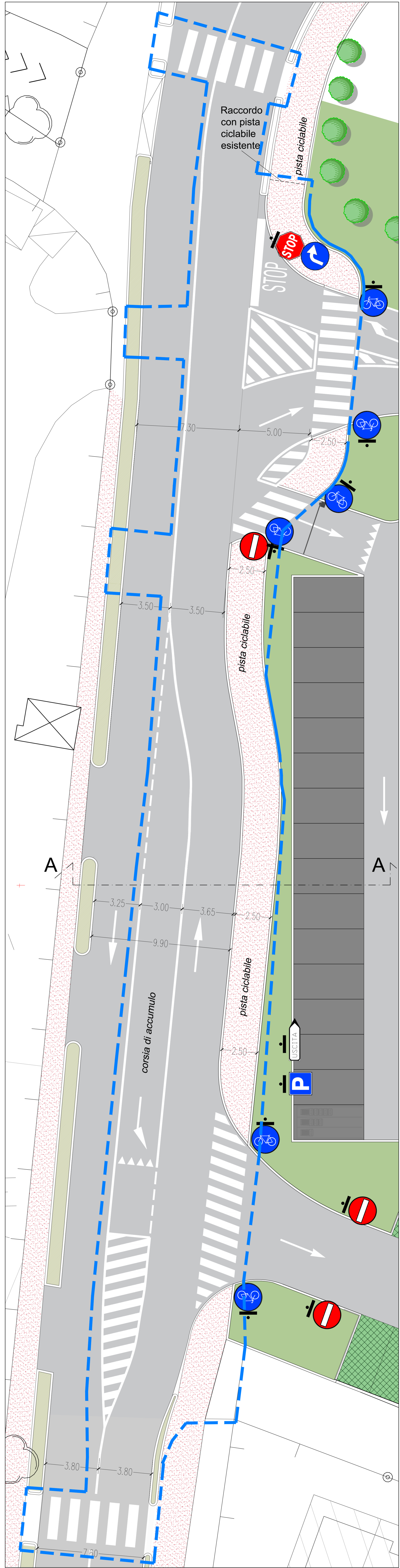
PLANIMETRIA DI PROGETTO
