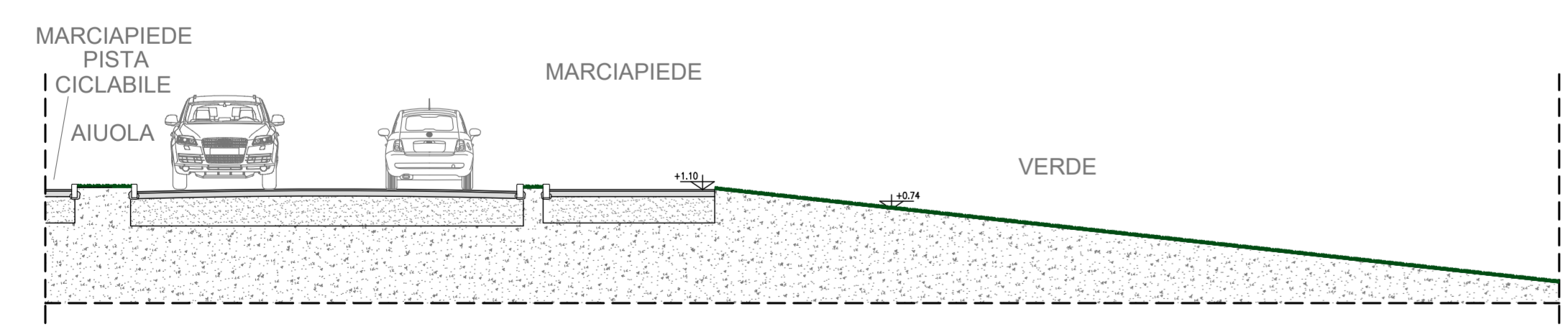
SEZIONE A-A STATO DI FATTO
