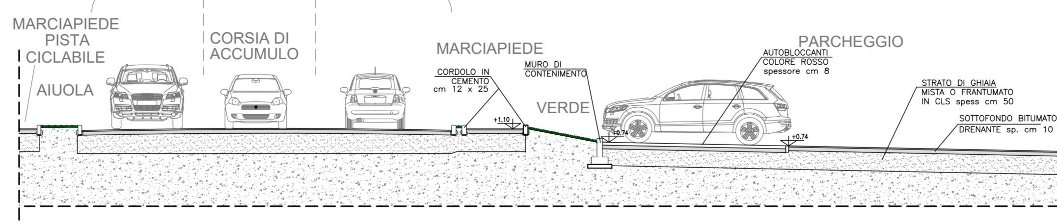
SEZIONE A-A DI PROGETTO
